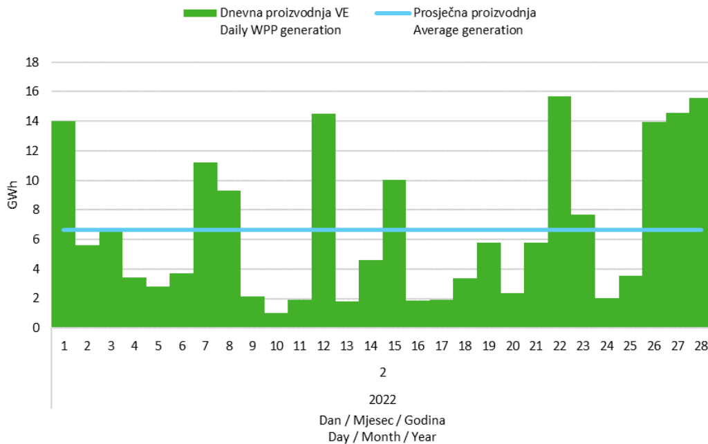
Slika 5 Dnevna proizvodnja svih vjetroelektrana u veljači 2022. godine Figure 5 Daily generation of all wind power plants in February 2022
