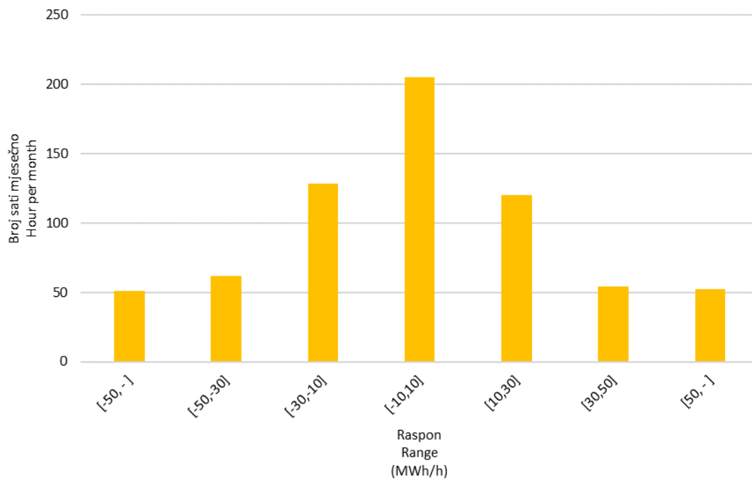
Slika 10 Statistička raspodjela satnih promjena proizvodnje VE u veljači 2022. godine
