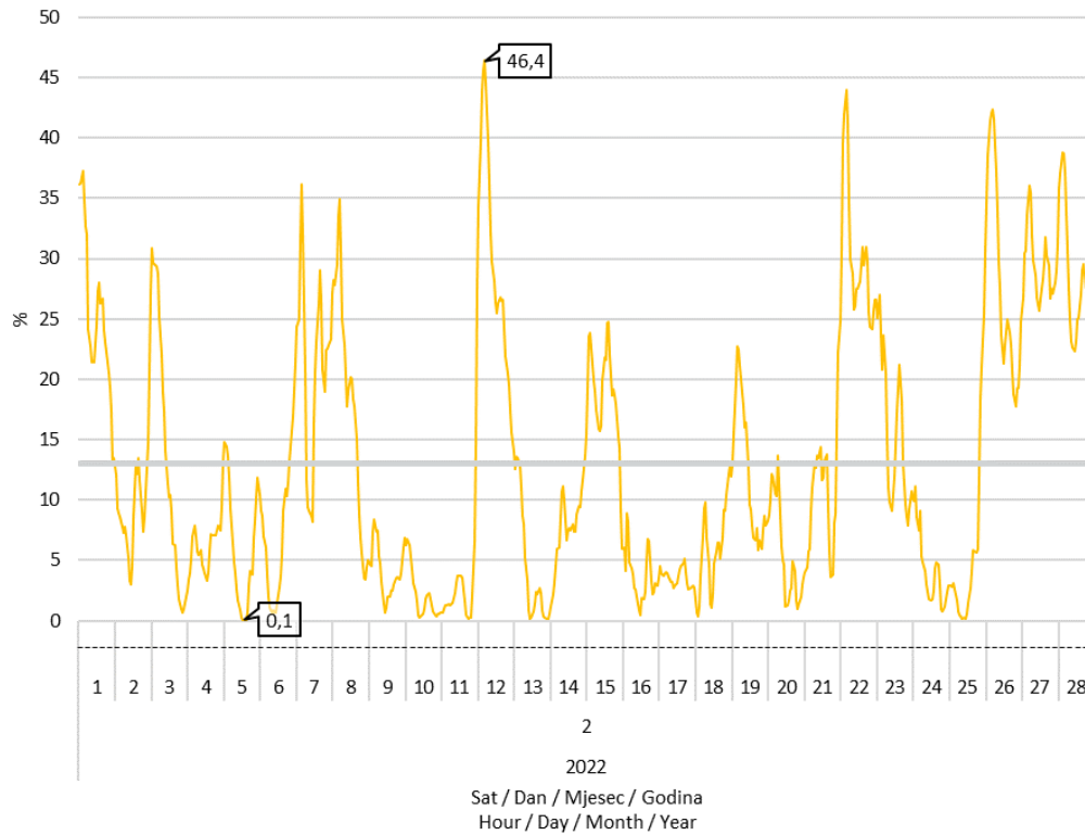
Slika 8 Udio proizvodnje vjetroelektrana u pokrivanju satnog opterećenja elektroenergetskog sustava u veljači 2022. godine
