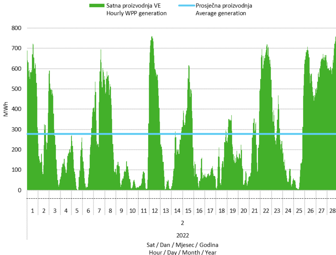
Slika 2 Satna proizvodnja svih vjetroelektrana u veljači 2022. godine Figure 2 Hourly generation of all wind power plants in February 2022
