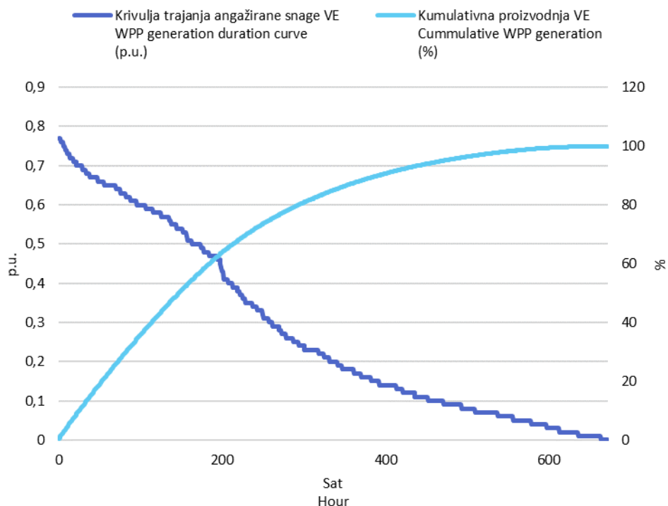
Slika 3 Krivulja trajanja angažirane snage svih VE i kumulativna proizvodnja VE u veljači 2022. godine u jediničnim vrijednostima
