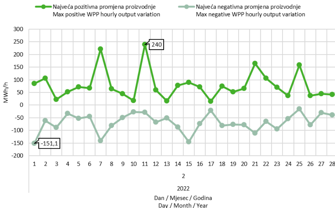
Slika 9 Maksimalna pozitivna i maksimalna negativna promjena satne proizvodnje VE u veljači 2022. godine
