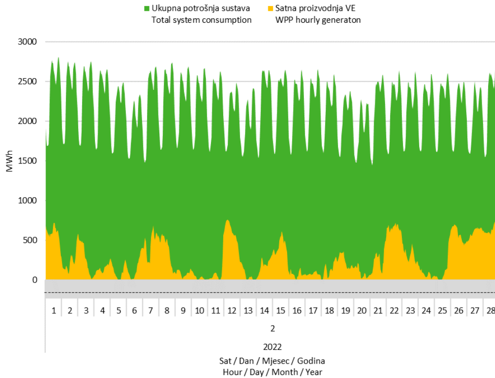
Slika 7 Usporedba satnog dijagrama opterećenja sustava i proizvodnje vjetroelektrana u veljači 2022. godine
