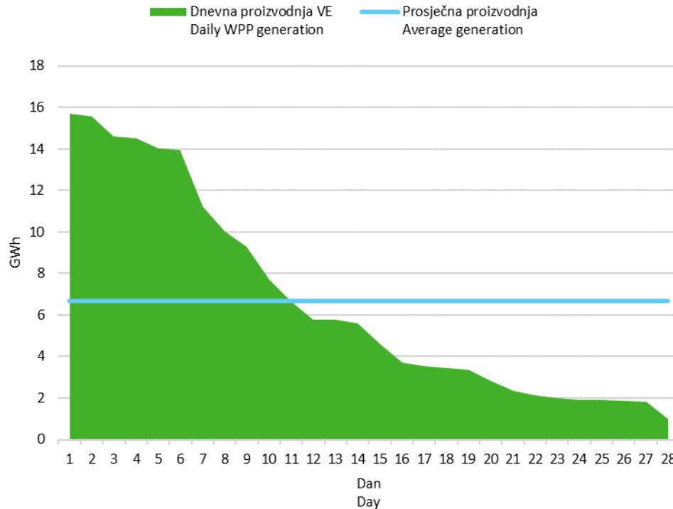
Slika 6 Krivulja trajanja dnevne proizvodnje vjetroelektrana u veljači 2022. godine
